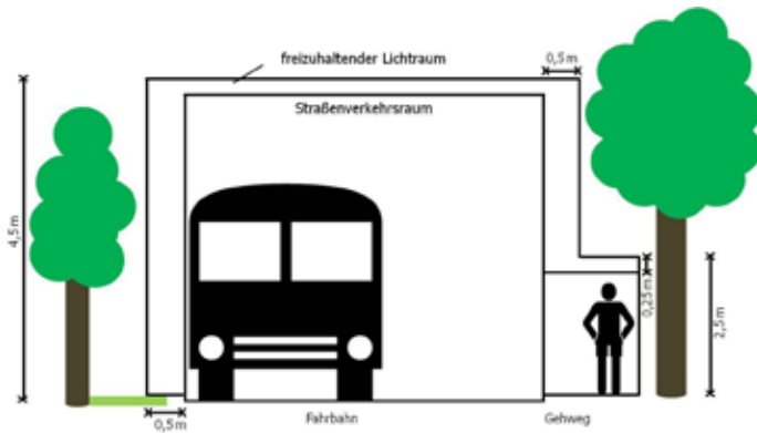
Straßenlichtraumprofil, das von Bewuchs freizuhalten ist
