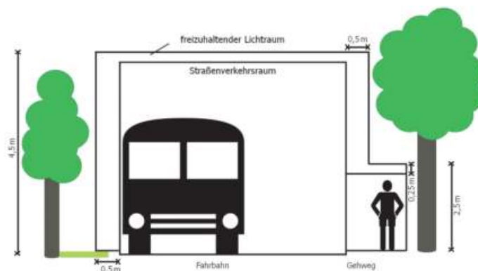
Grafik: Straßenlichtraumprofil, das von Bewuchs freizuhalten ist
